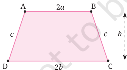
Fig. 6.29: Isosceles trapezium
